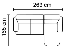
071 SECT.(16+49)
